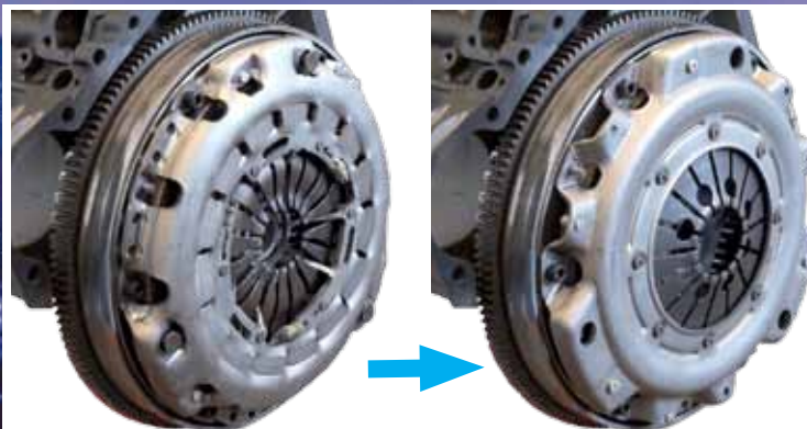
Sprzęgło samonastawne (SAC)
