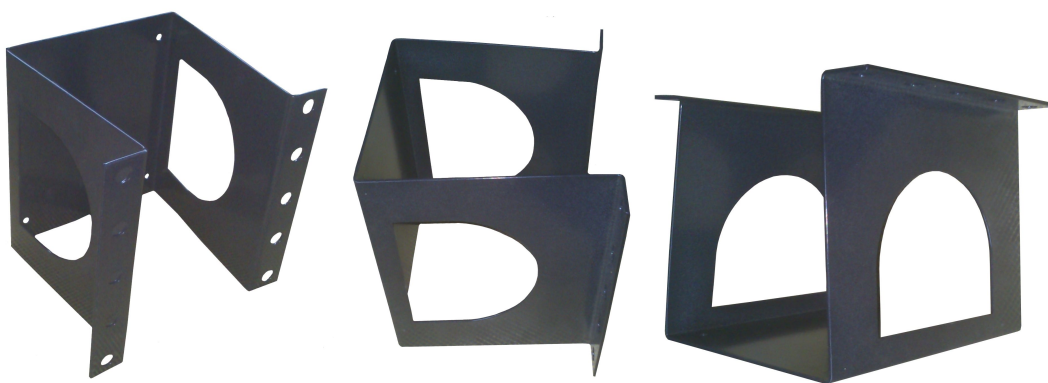
Uchwyt na plastikową skrzynkę na gaśnicę malowany proszkowo na kolor czarny Nr Vanstar: 107075R
